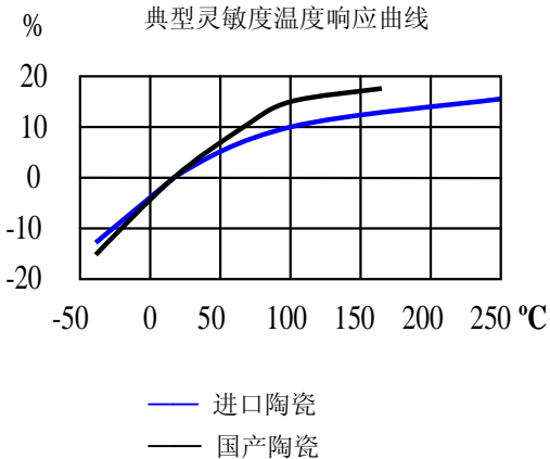
典型灵敏度温度响应曲线
