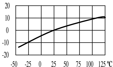
典型灵敏度温度响应曲线
